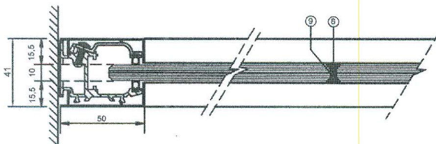
Οριζόντια τομή / Horizontal section
