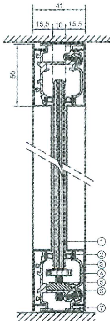
Κατακόρυφη τομή / Vertical section
