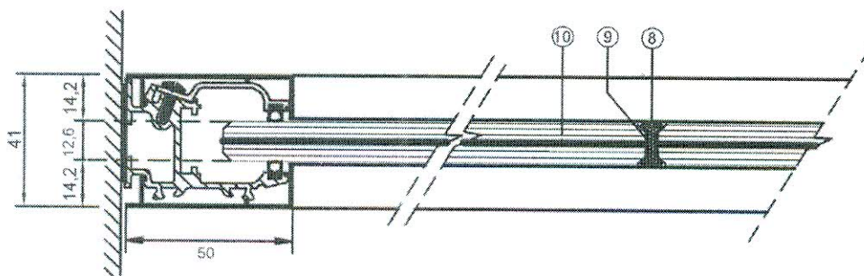
Οριζόντια τομή / Horizontal section
