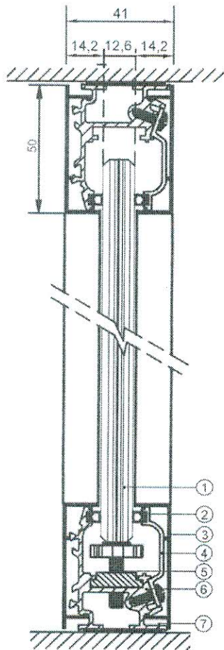
Κατακόρυφη τομή / Vertical section
